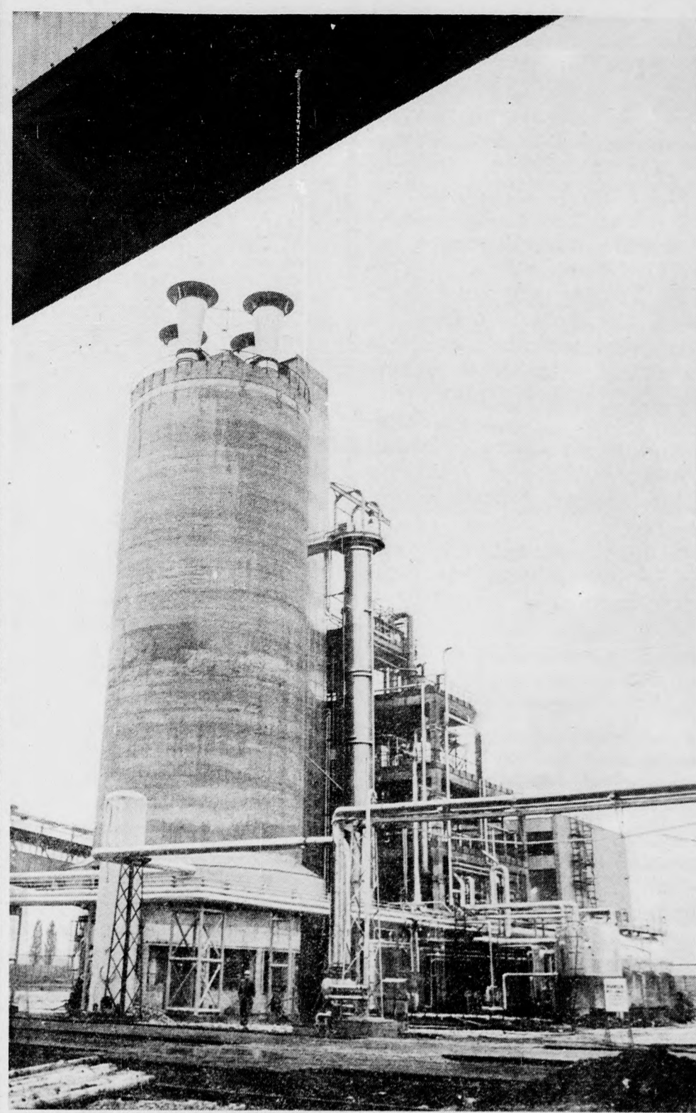
A kiemelt beruházások sorában is a fontosabbak közül való a Borsodi Vegyi Kombinát karbamid üzemé. Az új gyár a múlt évben már teljes kapacitással termelt, gyártmányaival importot takarít meg a népgazdaság. Távoli kép a karbamid üzem tornyáról.
