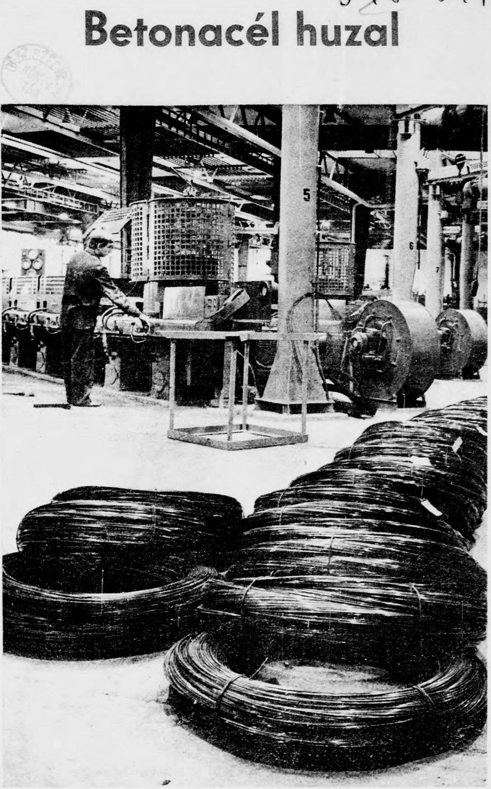
260 millió forint felhasználásával bővítették a Miskolci December 4 Drótműveket. Az új gyáregységben az építőiparban nélkülözhetetlen nagyvilárlású betonacél huzal gyártása folyik. A magyar, svéd és angol gyártmányú célgépekkel felszerelt üzem a teljes hazai szükség- letet kielégíti.
