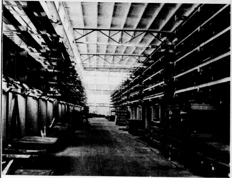
A Vörös Csillag Traktorgyár rekonstrukciója folyamán korszerű üzemek és berendezések kerülnek átadásra. Próbauzemelés alatt áll az „Aichelin” osztrák cég által szállított hőkezelő berendezés. A 3600 négyzetméter alapterületű vasraktárt, a daraboló üzemcsarnokot és a tanműhely épületét nemrég adták át rendeltetésének. Képfőnök: a traktorgyár új vasraktára. Az eddigi szabadban való tárolás helyett a legkorszerűbb tárolási és anyagmozgatási technológiát vezették be (MTI-fotó — Balassa F. felv.)
