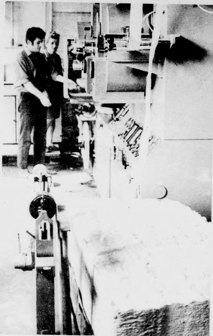
Filterrudgyártó gépsor
