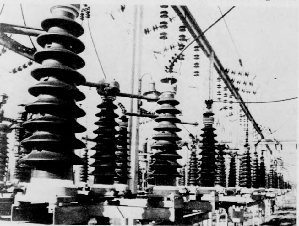
Porcelán szigetelők erdeje az állomáson
