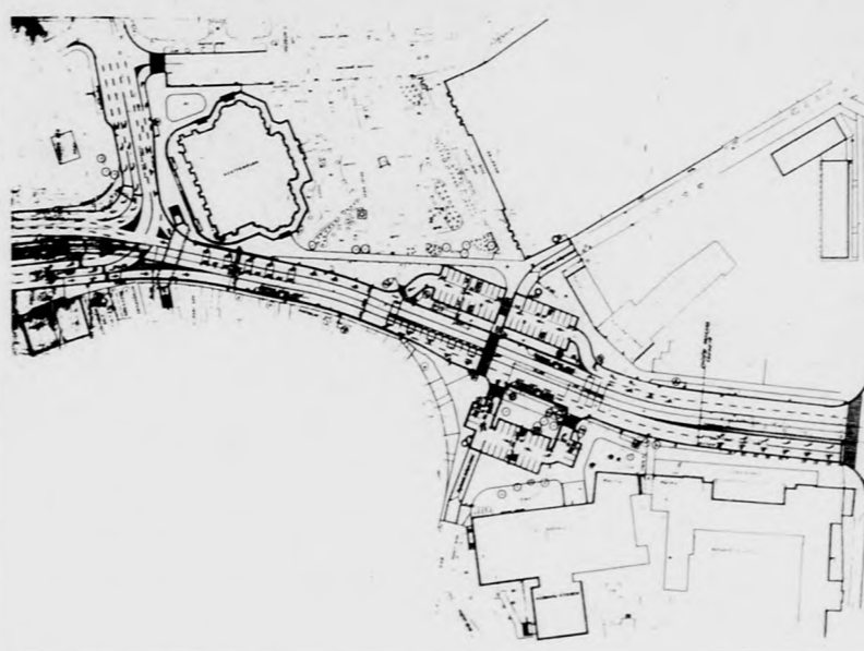
A Kálvin tér korszerűsítési terve (Készítette a Debreceni Tervező Vállalat)
