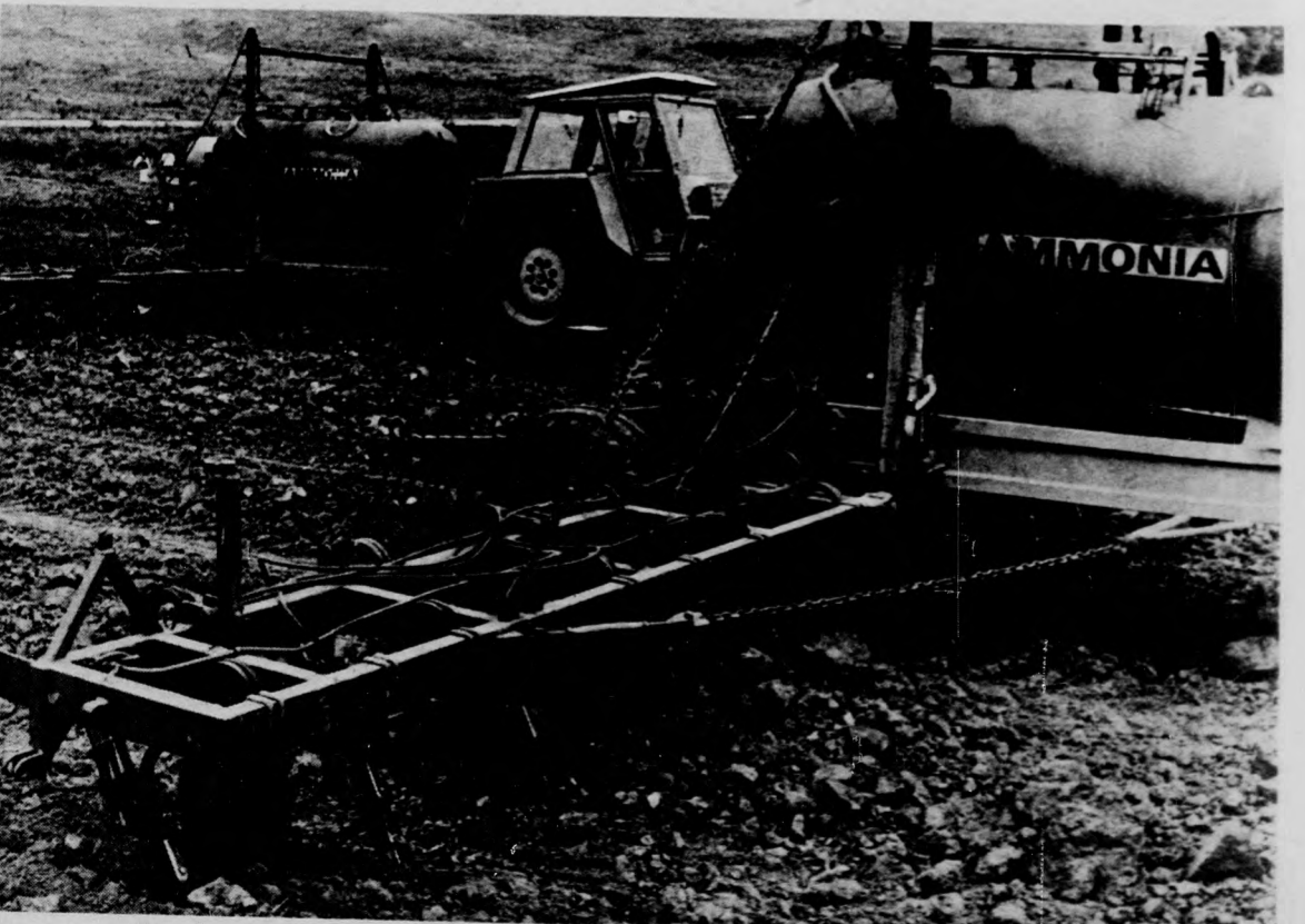
A dán gyártmányú injektáló gépek évente 16 ezer hektáron „terítik” az ammóniát
