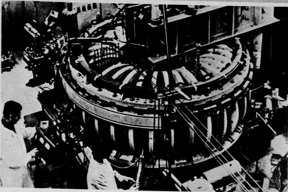
A szabályozott termonukleáris fúzió kísérleti berendezése a moszkvai Kurcsatov Intézetben (MTI Külföldi Képszolgálat — KS)
