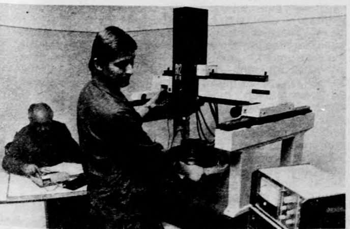
A Forgácsolószerkezeti Vállalat az idén több mint hatszázmillió forint értékben készít forgácsolószerkezeteket. A vállalat termékeinek egy részét a tőkés piacon értékesítik. Képeinken: Háromdimenziós mérőgépen ellenőrzik az exportra kerülő marófejeket
