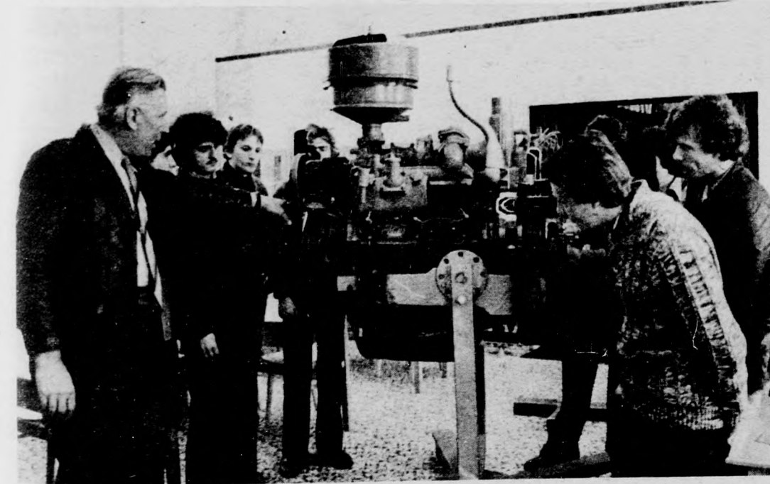
Bárdos László adjunktus T-150 K motorjának vízűtéses rendszerét magyarázza a diákoknak
