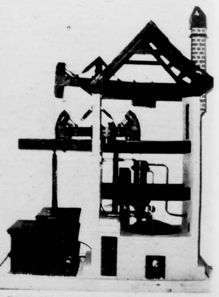
Egy tüzgép a 18. század elejéről (modell) (Szűk Ödön felvételei — KS)
