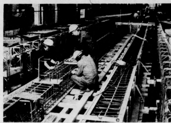
A MÁV Debreceni Járműjavító Üzemének új csarnokában a kilencedik vágány szintartó talpgerendáit szerelik az építők
