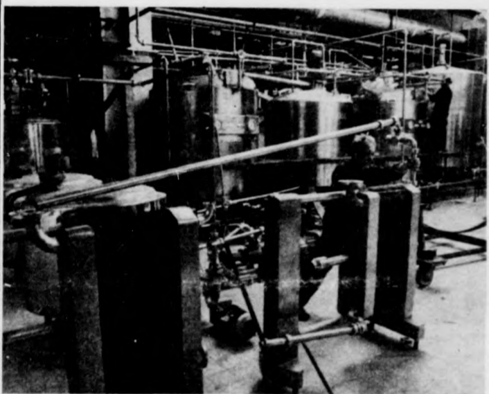
Rozsdamentes anyagból készült vezetékeken szállítják a tejet. A vezetékeket és a tartályokat az ÉLGEP szerelői állítják össze
