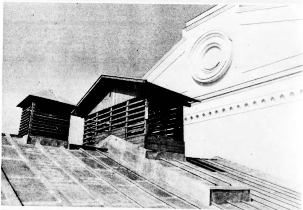
Elkészült a tetőszerkezet. Képünkön az új szellőzési rendszer egy részlete látható
