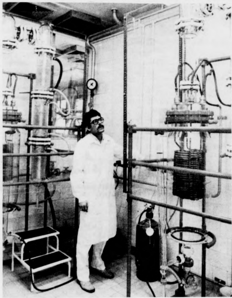
A desztilláló berendezés működés közben (Fotó: Iklódy János)
