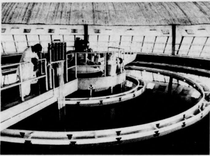
A víztisztítómű egyik derítője, ahol már csaknem látható a víz minőségű a víz
