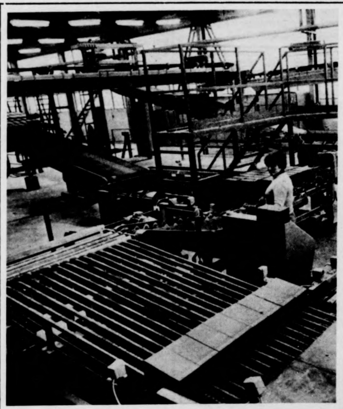
Az Épületkerámia-ipari Vállalat Gyömrői úti Kerámia Téglyárában befejeződött a rekonstrukció. Ötvenegy millió darab jó hőszigetelő tulajdonságú téglát gyártanak majd (MTI-fotó — Balaton József)
