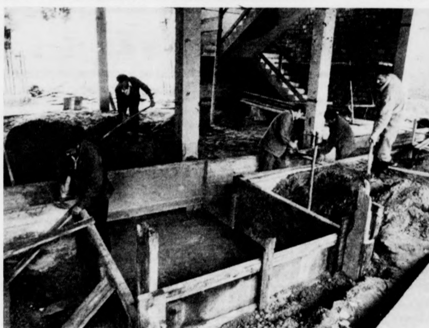
A műhelyterem betonozásán dolgoznak a munkások
