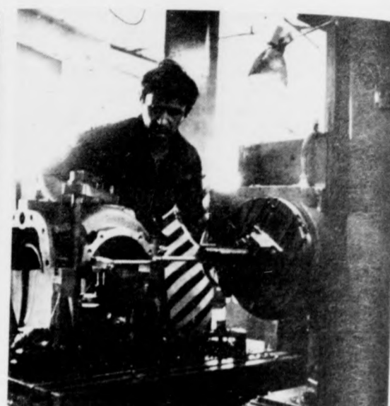
Vasforgácsok repülnek, formálódik a hajtóműház
