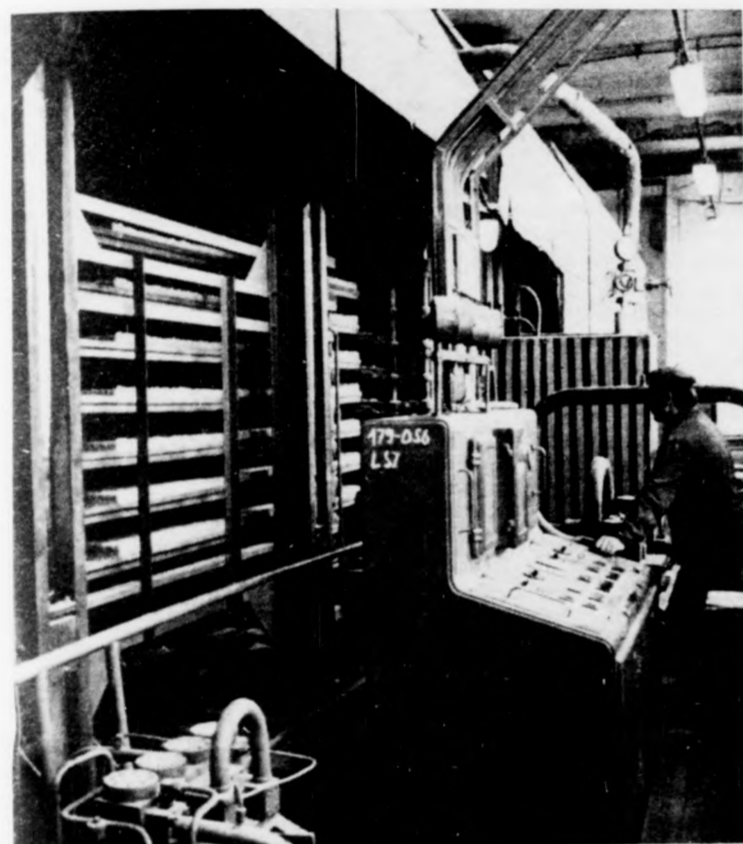
A feldolgozás során keletkezett pozdorjából bútorlapot gyártanak
