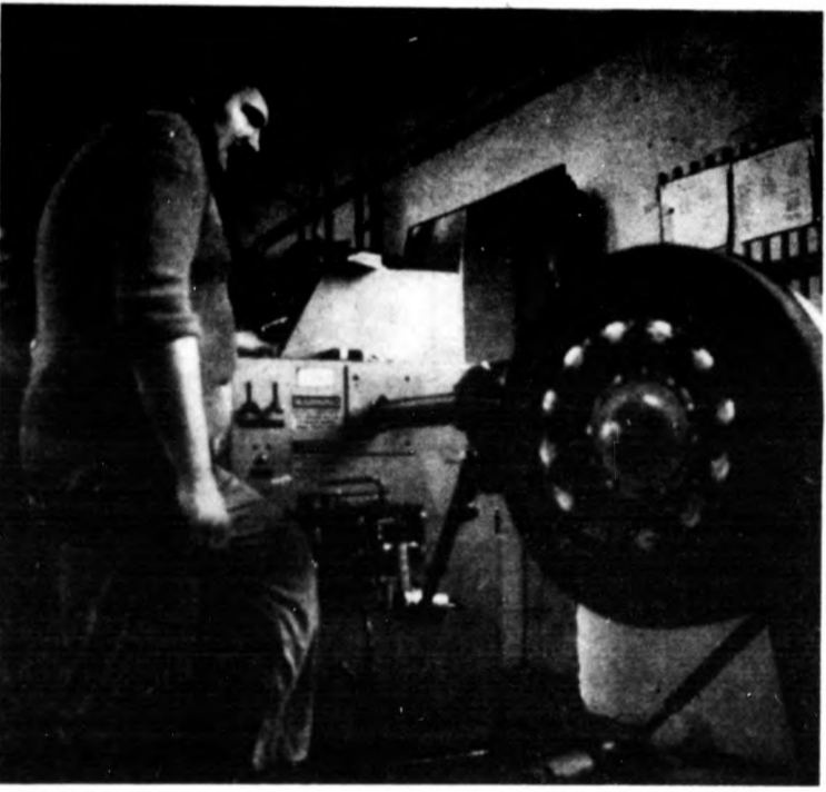
Képlékeny gumicsíkot visznek fel az abroncs felületére.
