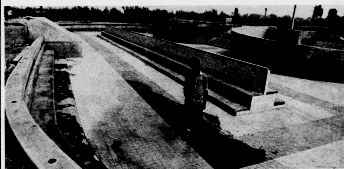
A melegvízes medence betonjának utókezelése
