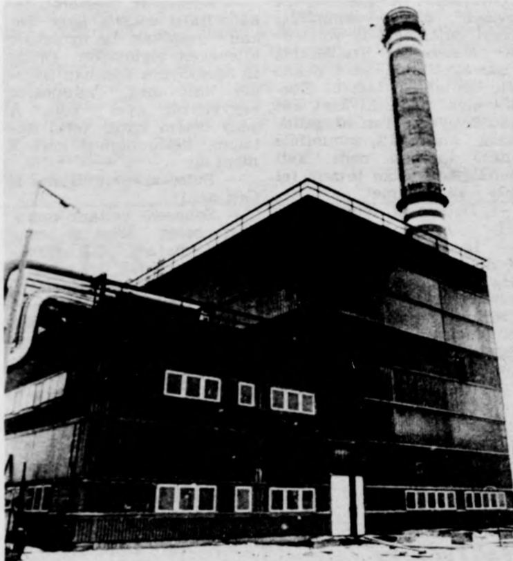
Az E50-40M típusú szovjet gőzkazán 50 tonna gőz fejlesztésére képes óránként. Képnél a gőzvezető csöveket szigetelik
