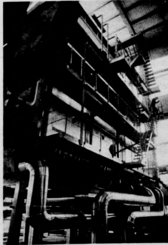
A szovjet KVGM-100-as típusú 116 megawatt teljesítményű forróvíz-kazán
