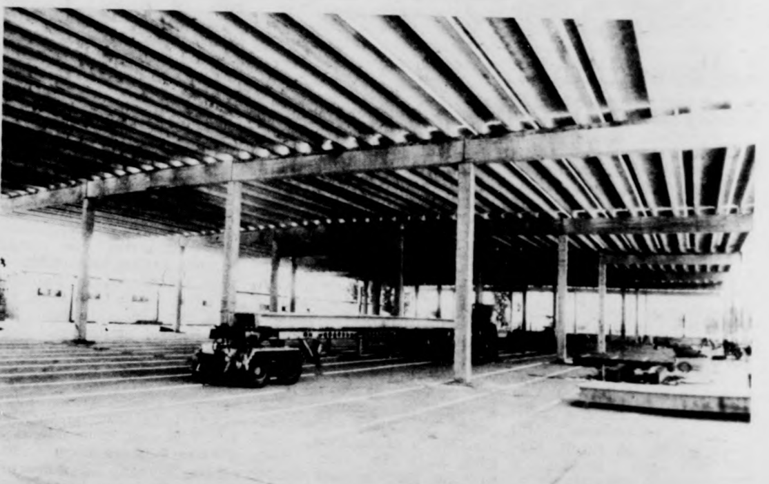
Készül a hűtőház a Konzervgyárban
