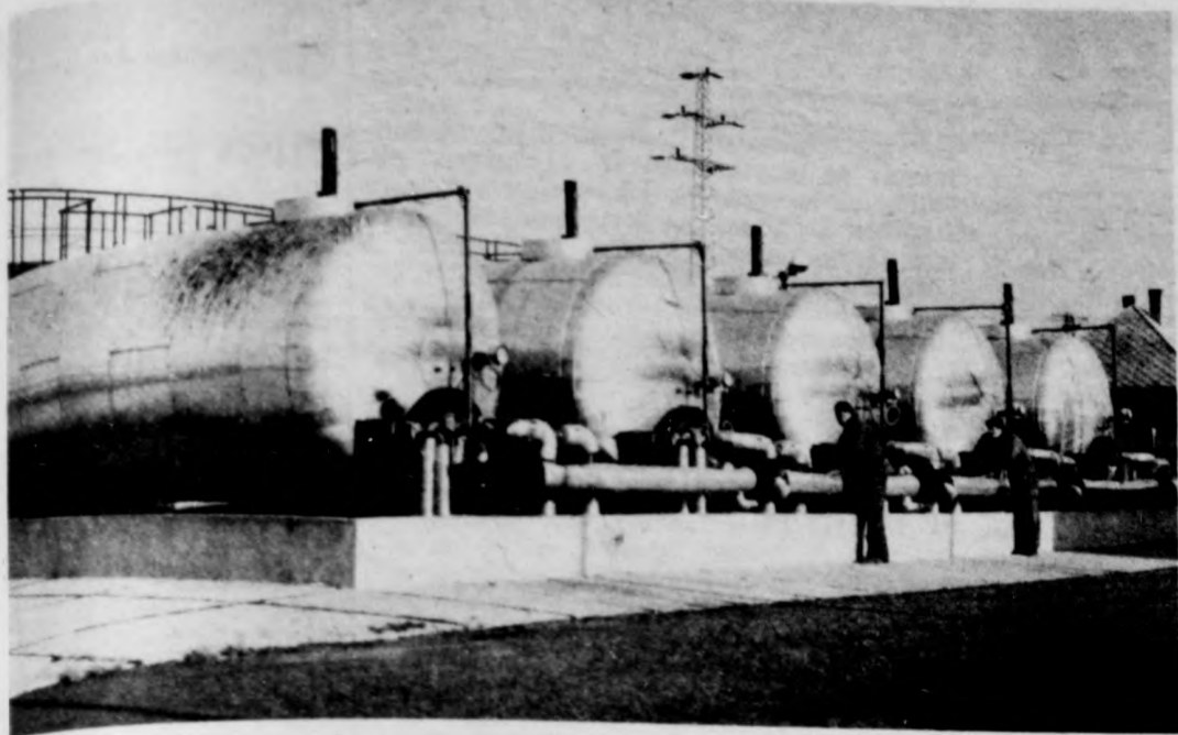
A bitumenemulziót gyártó üzemrész
