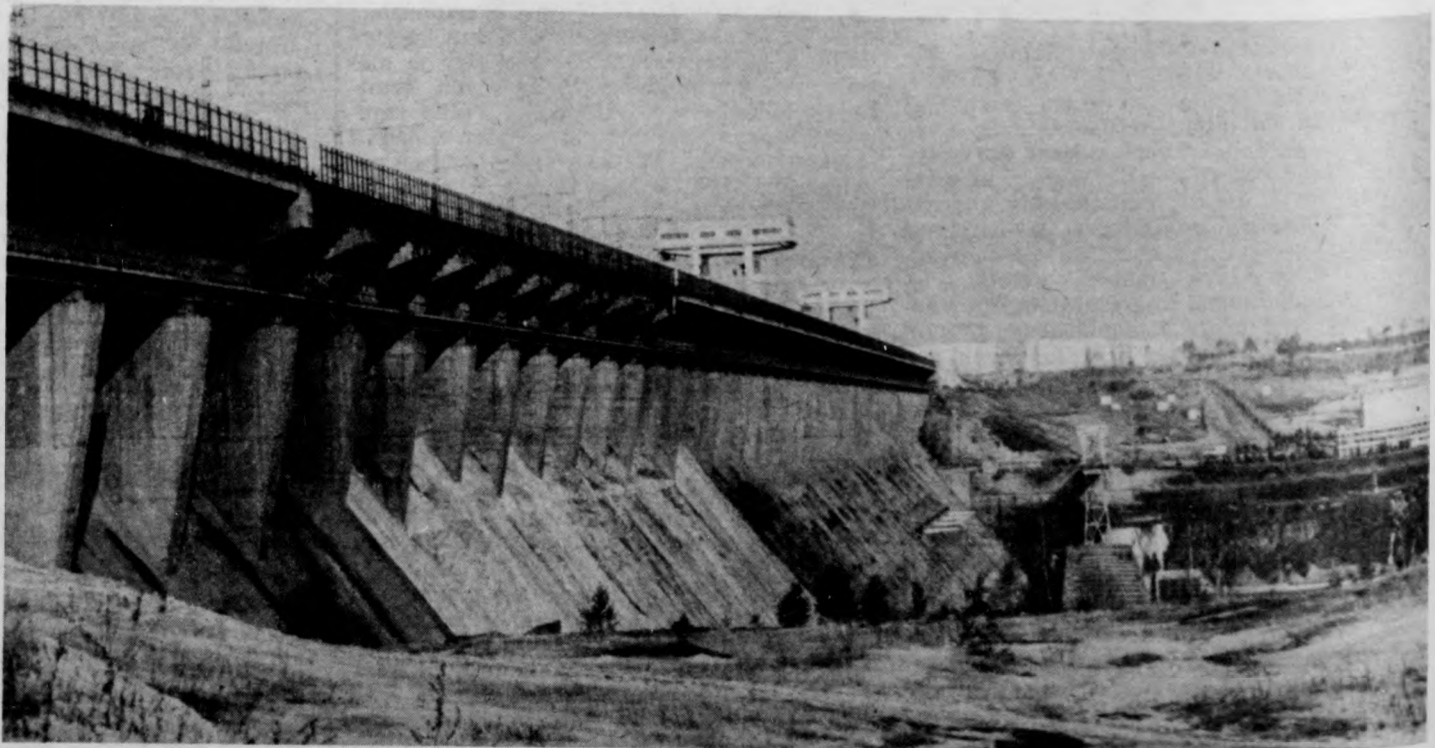
A BRATSKAI VÍZIERŐMŰ — KÉP ÉS SZÖVEG: ZOLTAI KÁROLY
