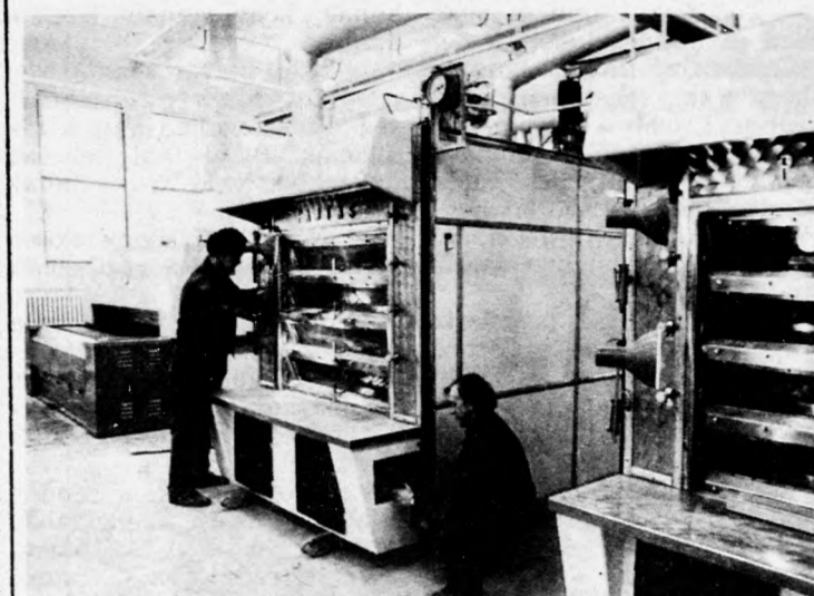
Az ÉSZKV már befejezte az új sütőüzem építését. Az 55 millió forint értékű beruházás a végső stádiumához érkezett, jelenleg a Csehszlovákiából érkezett gépek beszerelése folyik. Az új üzem kapacitása a jelenleginek másfélszerese lesz, tizenhat óra alatt tizenhat tonna kenyeret és péksüteményt képes előállítani
