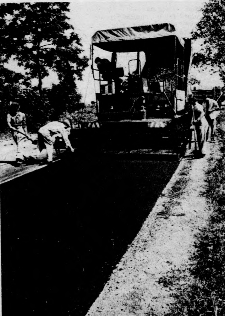
Az aszfaltozó gép naponta mintegy nyolcszáz méteres útszakasz aszfalttrétegét készíti el
