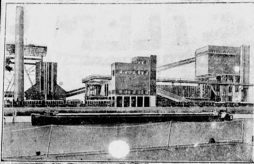
Felépült a világ legnagyobb kokszkályhája egy gelsenkircheni ipartelepen. A szakemberek a világ minden részéről özönlenek a technikai és építészeti csoda megtekintésére.
