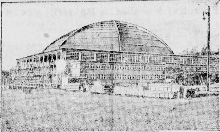
A világ legnagyobb kupolás építménye. A lipcei nagy vásárcsarnok. — A kupola átmérete 67 méter, felülete 6000 négyzetméter.
