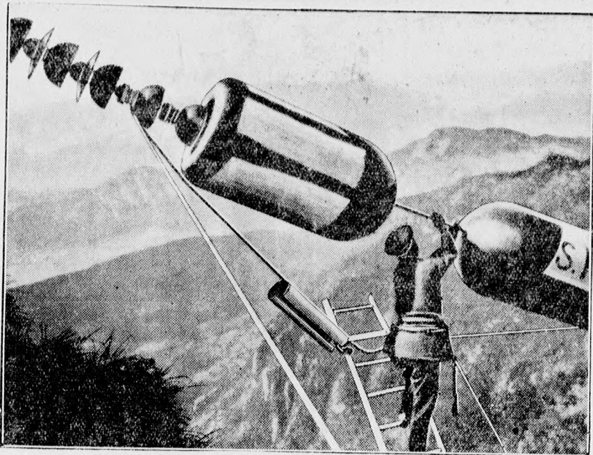
Szigetelő lánc villámfogás céljára a Monte Generoson. Német tudósok új energia források után kutattak és ennek során kísérleteztek azzal, hogy a villámban rejlő óriási villamos erőt igyekezzenek a cél szolgálatára megfogni.
