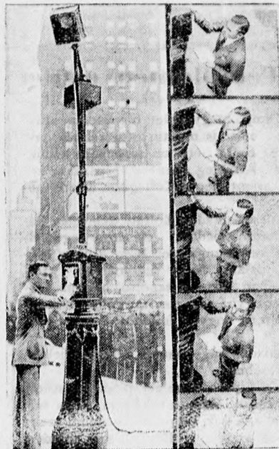
Walker newyorki polgármester kipróbálja az automatikus kamarával felszerelt legújabb tüzelő készüléket. Jobbról a tüzelő készülék fényképe. Newyorkban az új tüzelő készülékkel védekeznek a jókedvű alarmirozók ellen: a készülék rögtön lefényképezi azt, aki a jelzést adja és egyuttal éles szirénát szólal.
