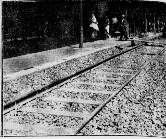
Vasbeton talapzatra raknak le sineket a debreceni pályaudvaron. A vasúti fatalpokat, amelyeket, annak ellenére, hogy impregnálva vannak, mégis csak ki kell az idők folyamán váltani, most az egész országban vasbeton talapzattal helyettesítik. A kicserélés fokozatosan megy, aszerint, amint valamelyes talapzat kicserélése szükségessé válik. A vasbeton talapzat kitűnően bevált. Képünk a sínlerakási munkálatokat mutatja be a debreceni pályaudvaron, valamint a vasbeton talapzaton fekvő már lerakott sínpar egy készen levő részét. (A Debreceni Független Újság felvételei.)
