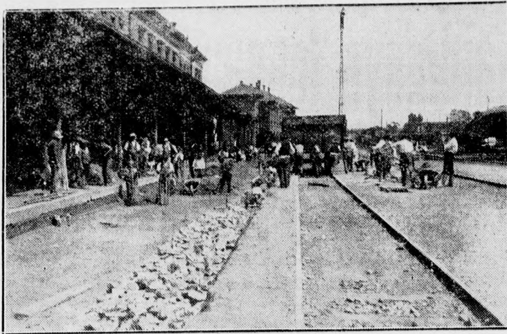
Vasbeton talapzatra raknak le sineket a debreceni pályaudvaron. A vasúti fatalpokat, amelyeket, annak ellenére, hogy impregnálva vannak, mégis csak ki kell az idők folyamán váltani, most az egész országban vasbeton talapzattal helyettesítik. A kicserélés fokozatosan megy, aszerint, amint valamelyes talapzat kicserélése szükségessé válik. A vasbeton talapzat kitűnően bevált. Képünk a sínlerakási munkálatokat mutatja be a debreceni pályaudvaron, valamint a vasbeton talapzaton fekvő már lerakott sínpar egy készen levő részét. (A Debreceni Független Újság felvételei.)
