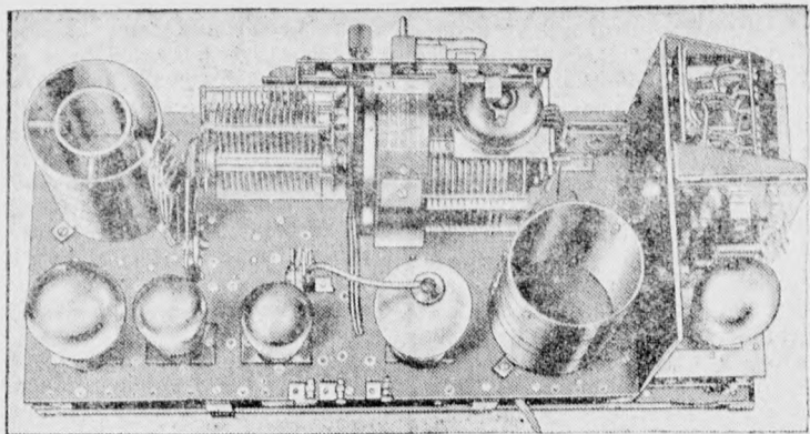
A most megnyílt rádió-kiállítás egyik nevezetessége, a legmodernebb Telefunken felvevőkészülék.
