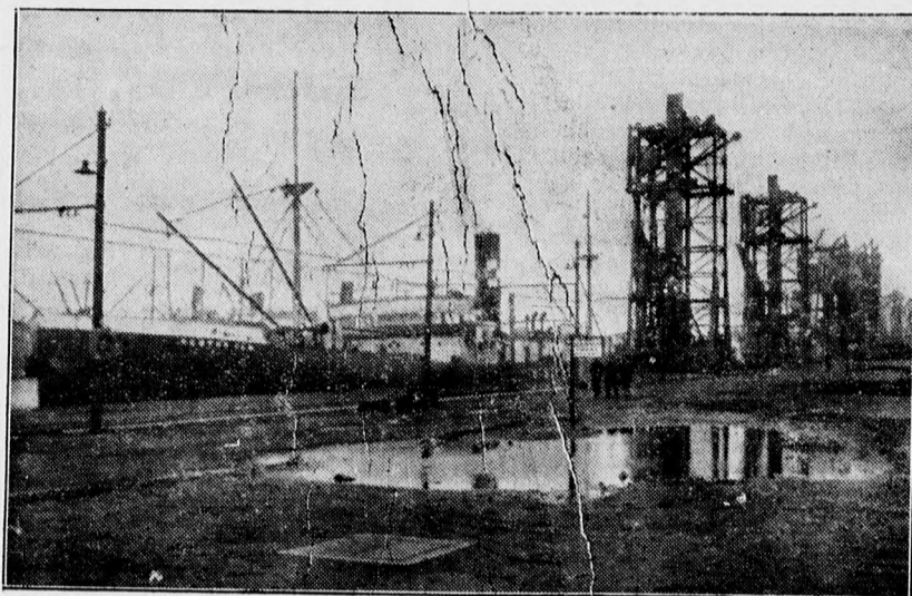
A szénkikötő Cardiffban. A hatalmas szénrakodódaruk egyszerre egész vagon szénen raknak a hajóba. (Debreceni János bányamérnök amatőr felvétele.)
