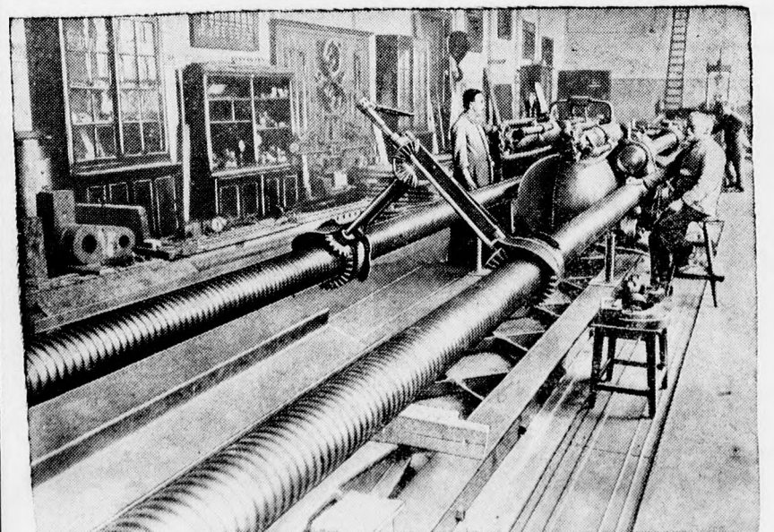
A dahlemi birodalmi anyagkísérleti állomás. A szakitógép, amely 500 tonnányi súlyig állapítja meg valamely tárgy ellenállási, vagy teherbírási erejét.
