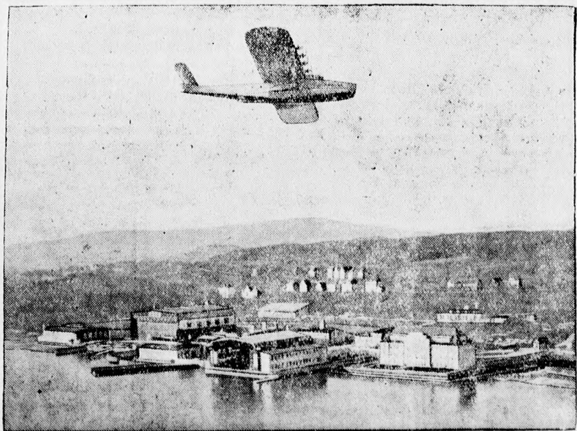
A „DO X” óriási repülőgép 169 utasával a bojeni tó felett 40 perces sikeres próbarepülésén, és a próbarepülésen 400 méter magasságban a repülőgép 12 motorja 6000 lóerővel dolgozik 170 kilométeres óránkénti sebességet ért el.
