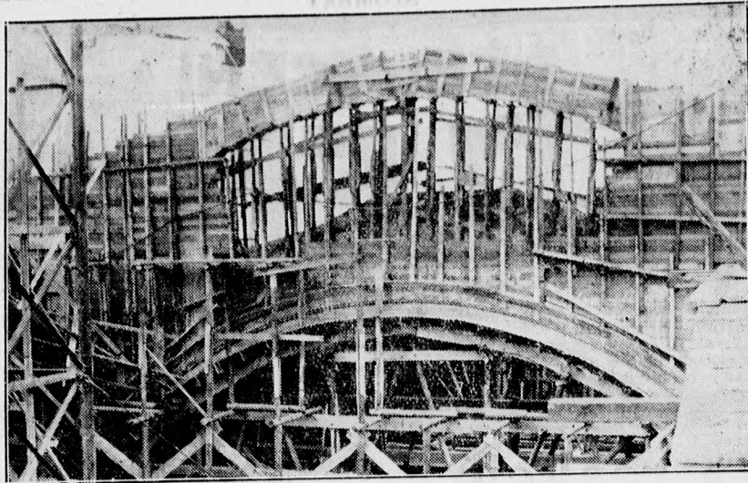
A debreceni Tisza István Tudományegyetem építkezése. — Érdekes íves dongás vasbeton szaluzási részlet. (Varga fényképész felvétele.)
