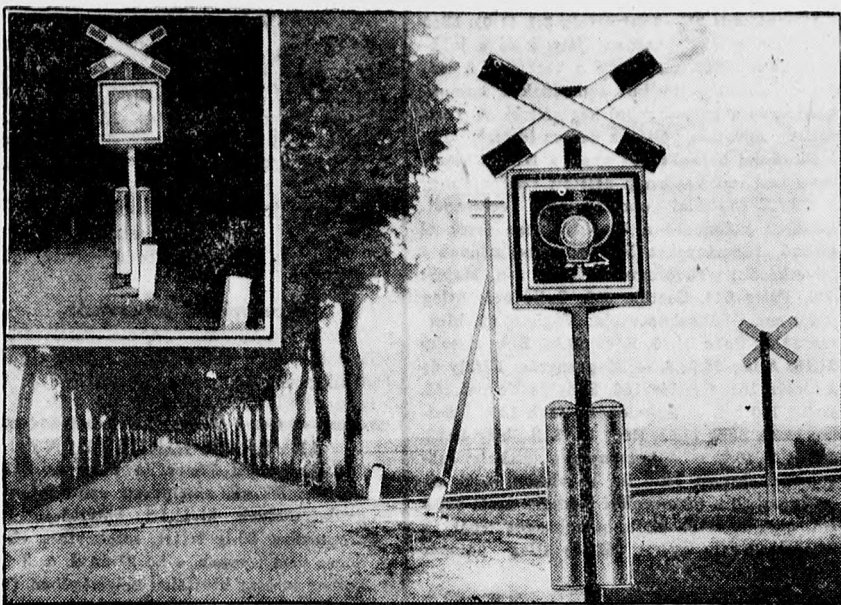
Kisérletezés fényjelző figyelmeztetővel a vasuti átjárónál. — Fenn a sarokban: A fényjelző készülék éjszaka működésében.
