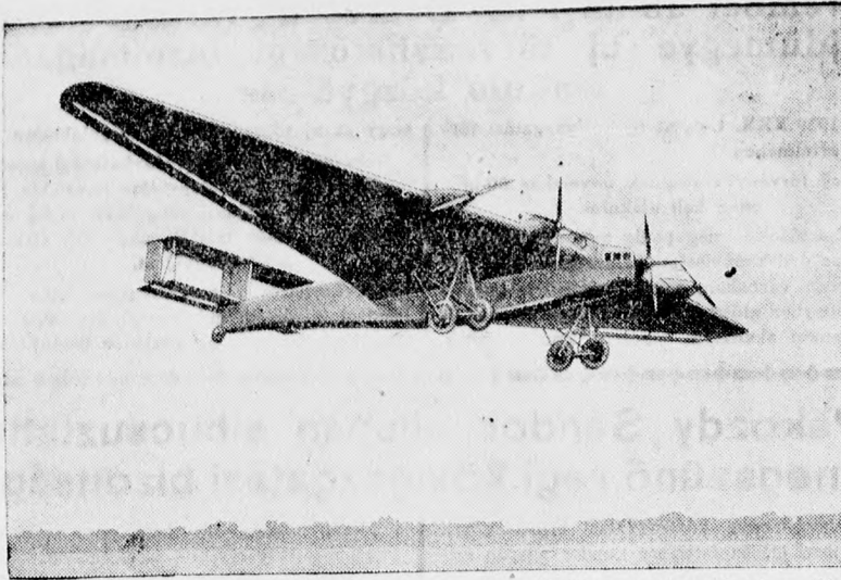
Az új Junker óriásrepülőgép, a G 38., amelyet a Repülő Ház-nak neveztek el, a világ legnagyobb repülőgépe. Dessau felett Zimmermann pilóta vezetésével most állotta ki a sikeres próbát. A repülőgép szárnyhossza 45 méter, a gép hossza 23 méter, motorjai összesen 2600 lóerejűek.
