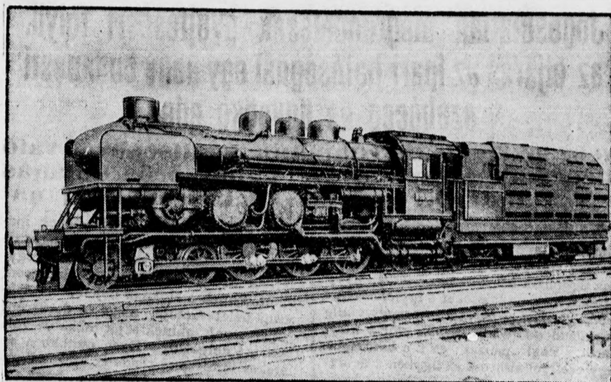
A német birodalmi vasutak új turbinás lokomotívja.
