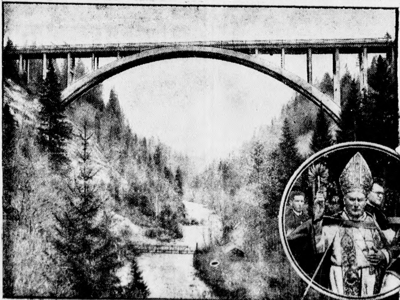
A 135 méter hosszú betonhid, 75 méter magasságban Eschelsbachnál, Oberammergau mellett, amelyet most avattott fel Faulhaber müncheni kardinális (a körben).
