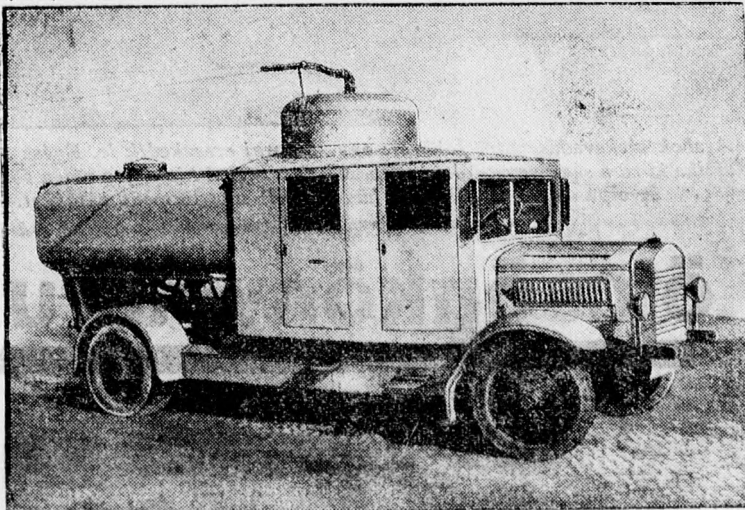
A berlini rendőrség vízfecskendő autója, amelyet a legutóbbi zavargásoknál is használtak a tüntető tömeg feloszlására. Az autó tartálya 5000 liter vizet fogad be és az autófecskendő vizsugarát 50 méterre veti.
