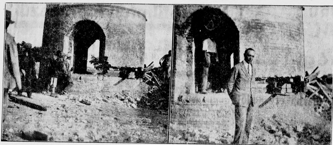
A városi téglagyár 40 méter magas régi kéményét ledöntötték. Jobbról: Az aláducolt kémény, előtte dr. Vida Szüts Imre városi főmérnök. Balról: A munkások meggyújtják a faducokat, amelyeknek kiégése után — egy óra elteltével — a kémény oldalra dőlt.
