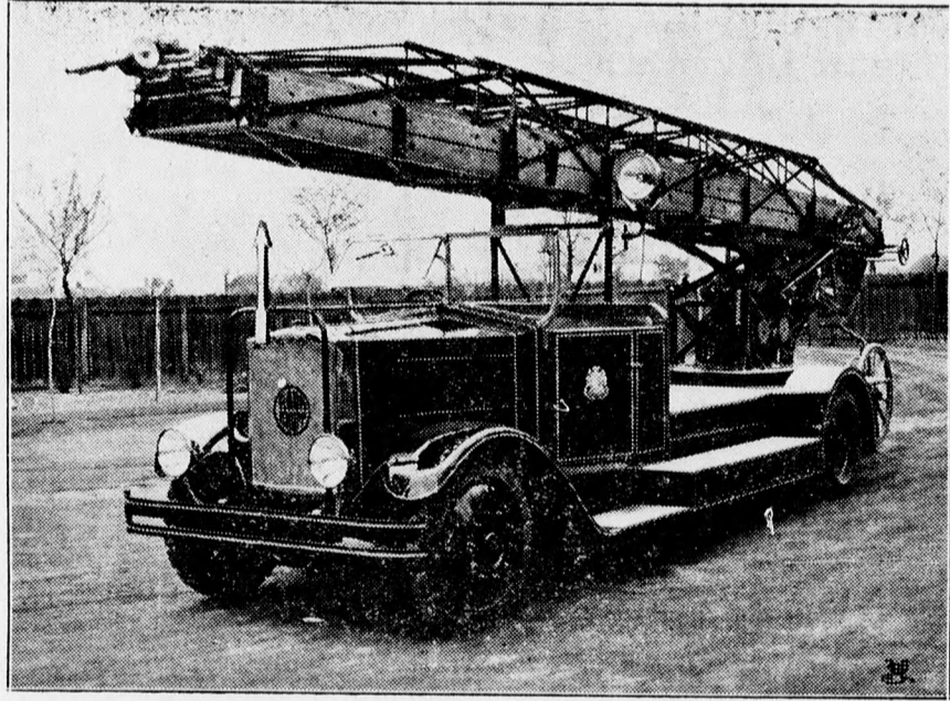
A Magyar Waggon és Gépgyár által a győri tűzoltóságnak szállított 28 méteres autotolólétra. — Ennek a testvérgépet rendelik meg a debreceni tűzoltóság számára.
