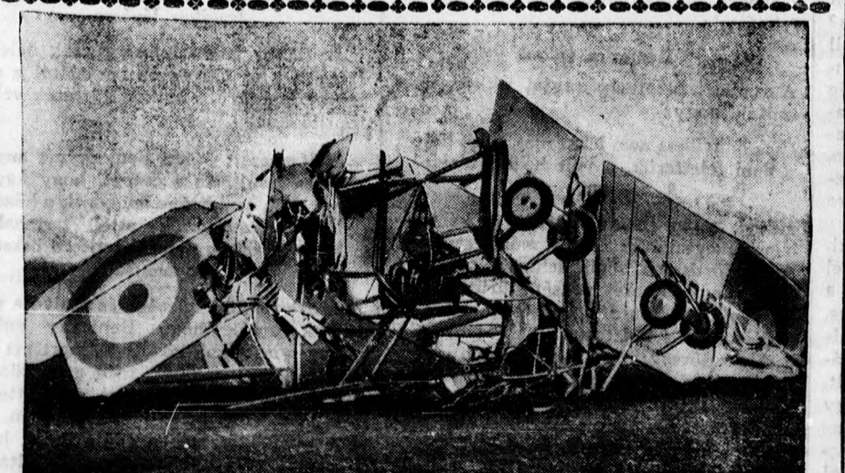
Gyakorlatozás közben a levegőben összeütközött két angol repülőgép romjai. — Két tiszt és egy altiszt meghalt.
