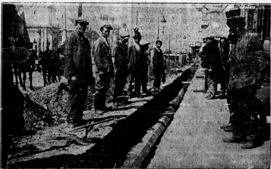
A főposta előtti kábel vezetéket fel kellett cserélni, mert az évek során elgörbült. Képünkön a napvilágra hozott kábel hullámvonalaszerű görbülései láthatók.
