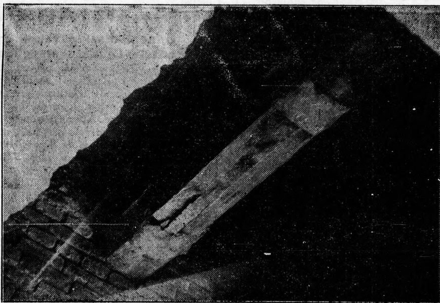
A Dobozy átjáró előtti résznek már valósággal törés lett a kábel görbülésének következménye.
