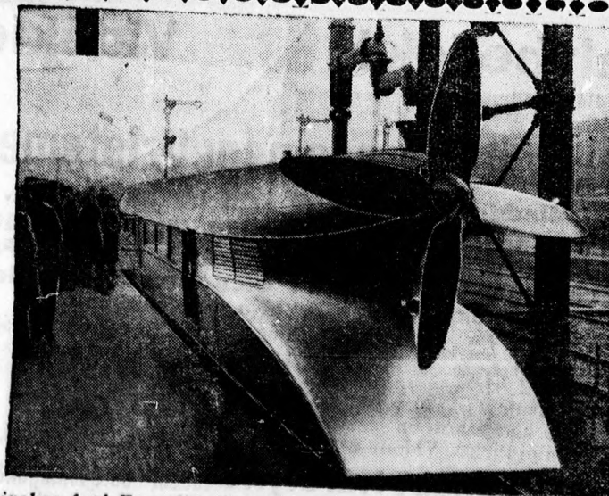
A sineken futó Zeppelint átadták a forgalomnak. — Képünk a Zeppelint indulás előtt a hannoveri pályaudvaron mutatja.
