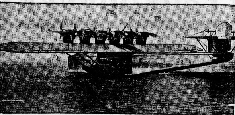
A Do. X. II. óriásrepülőgép a spézi kikötőben, Olaszország legnagyobb hadikikötőjében, ahová a Dornier-művek altenearei telepéről repült két óra alatt az Alpok felett. Az óriás gépet a német cég az olaszok részére építette.
