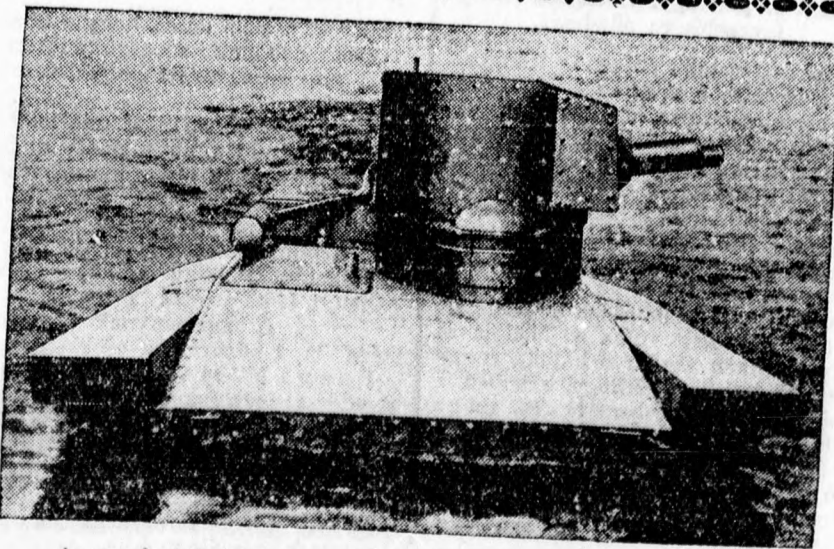
Az angol új óriási tank, amely folyókat és tavakat is át tud szelni.
