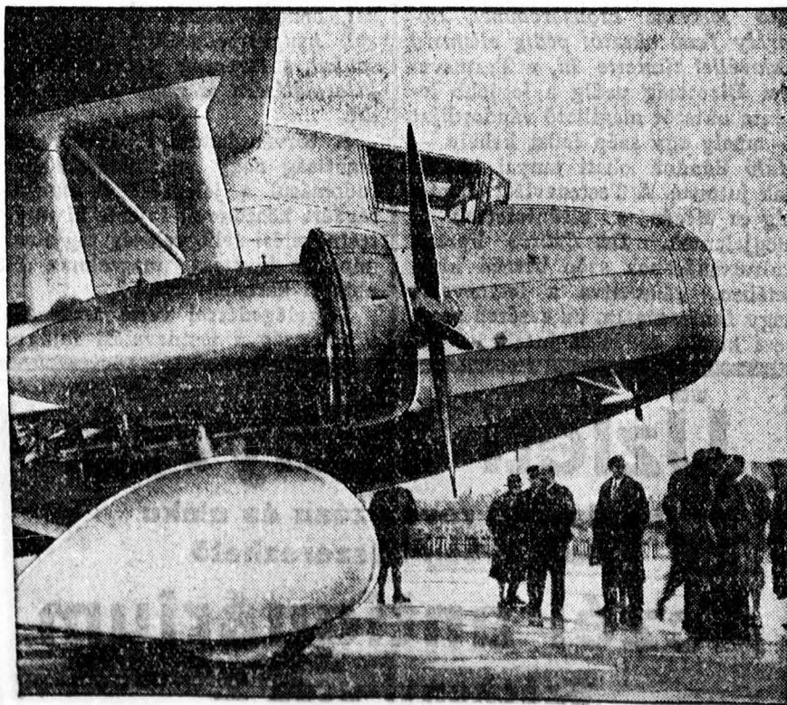
A „Do X”, a Dornier-művek új alkotása a Berlin—Tempelhof repülőtéren, ahová Friedrichshafenből érkezett meg. A négymotoros óriási gép, amely 10 utast szállít, a gyors közlekedésre van berendezve, Stuttgart és Berlin között az utat két és fél óra alatt teszi meg.
