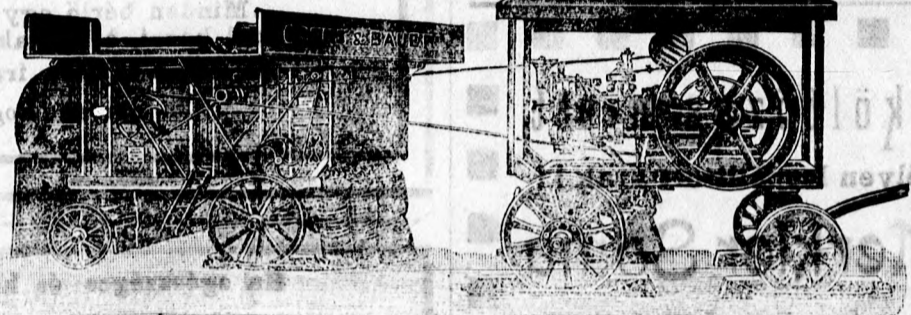
Benzin-lokomobil. — Szivó-gázmotor.
